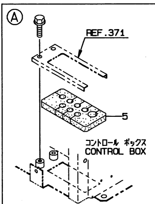
パイプ ホルダー 部詳細 DETAIL OF PIPE HOLDER
