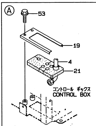
パイプ ホルダー 部群集 DETAIL OF PIPE HOLDER
