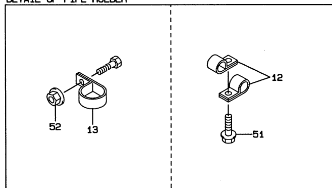
パイプ ホルダー 部群集 DETAIL OF PIPE HOLDER
