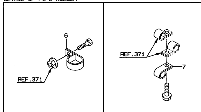
パイプ ホルダー 部詳細 DETAIL OF PIPE HOLDER
