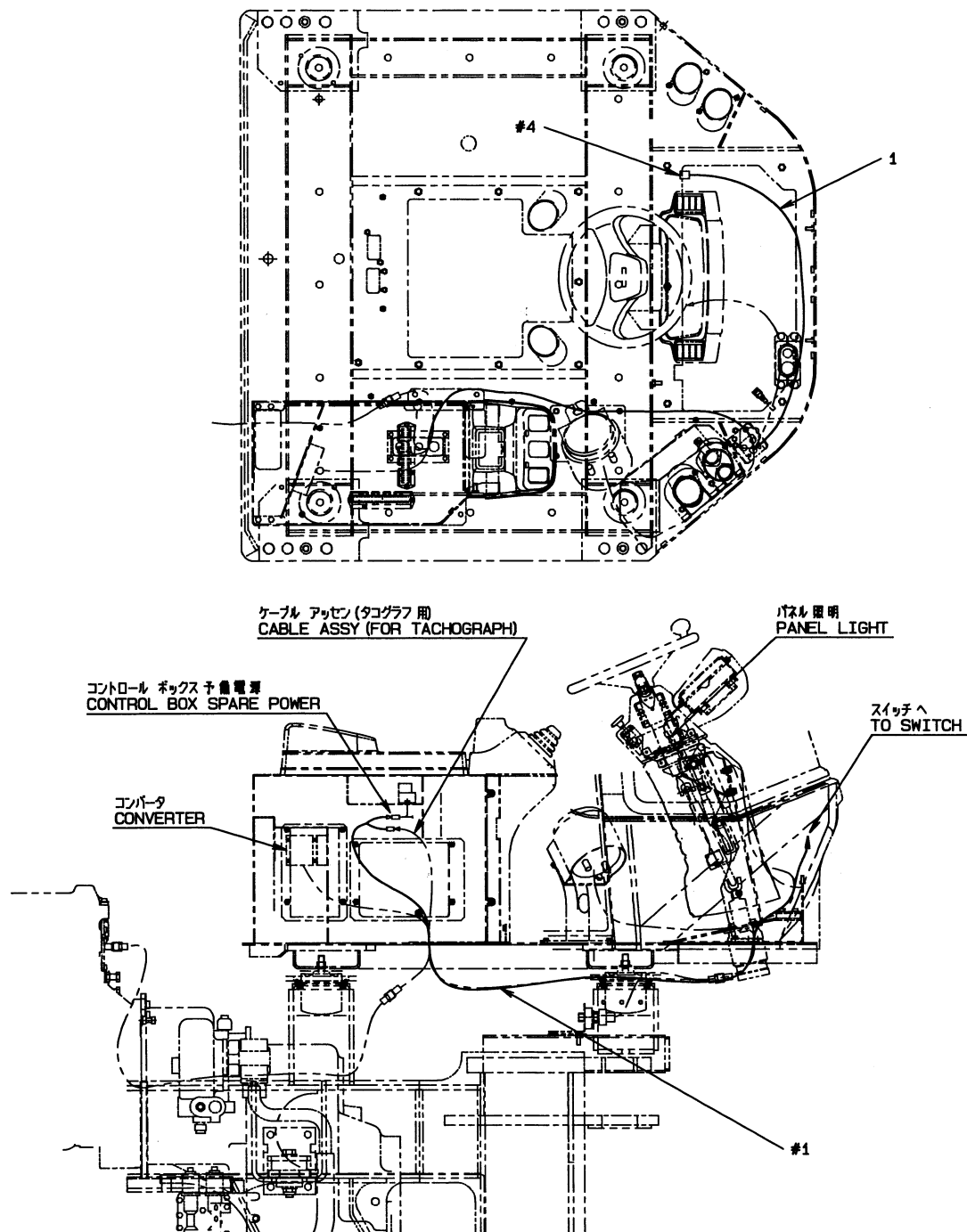
スイッチ ボックス 部詳細 (キャブ) DETAIL OF SWITCH BOX (CAB)
