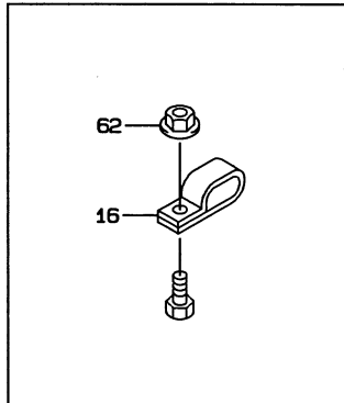
パイプ ホルダ 部群 DETAIL OF PIPE HOLDER
