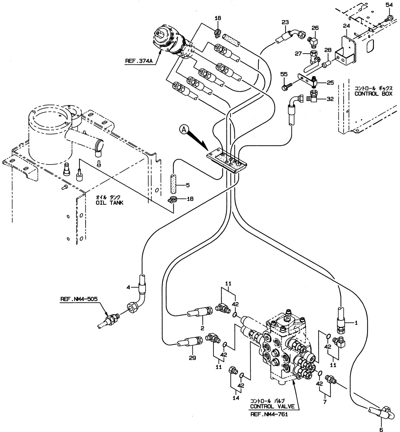
パイプ ホルダー 部群集 DETAIL OF PIPE HOLDER
