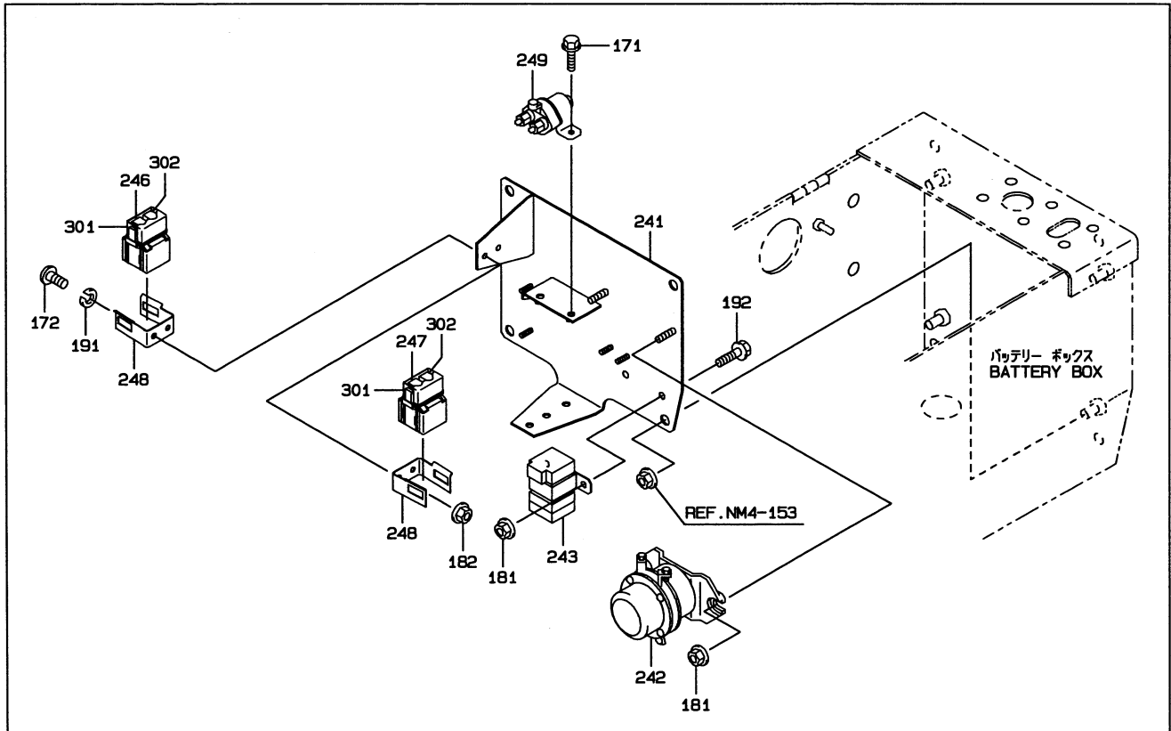
リレー ユニット マウント RELAY UNIT MOUNT
