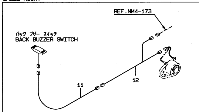
ケーブル マウント CABLE MOUNT
