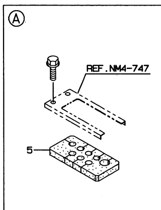
パイプホルダ部詳細 DETAIL OF PIPE HOLDER
