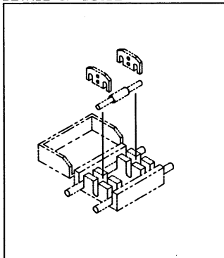
ダイオード 部詳細 DETAIL OF DIODE
