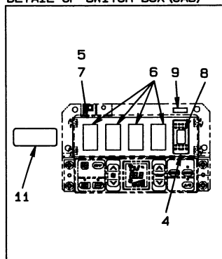
スイッチ ボックス 部詳細 (キャブ) DETAIL OF SWITCH BOX (CAB)
