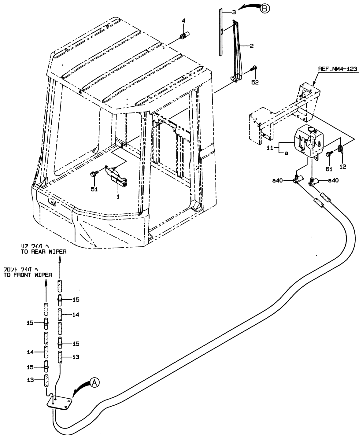
パイプ ホルダ 部群 DETAIL OF PIPE HOLDER
