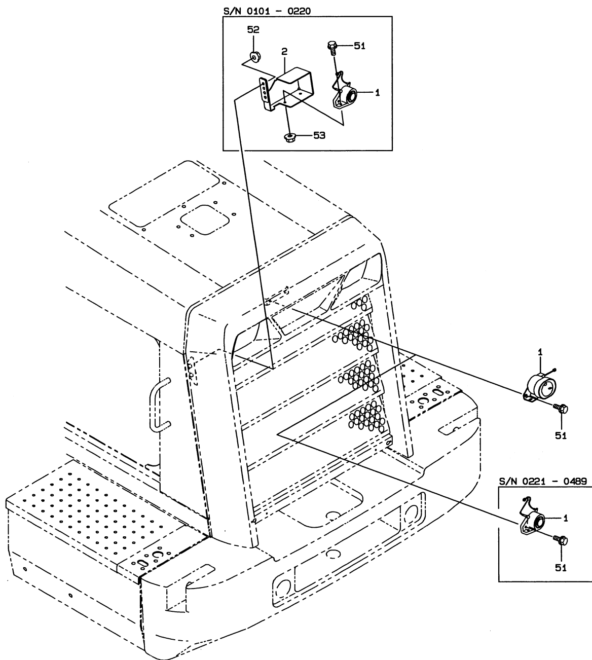
ケーブル マウント CABLE MOUNT
