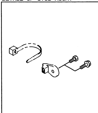
スタッド マウント 部 詳細 DETAIL OF STUD MOUNT
