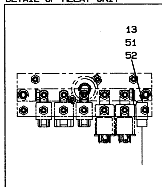
リレー ユニット 部詳細 DETAIL OF RELAY UNIT
