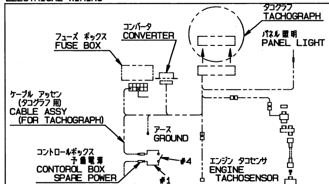
電気的 ワイヤリング ELECTRICAL WIRING
