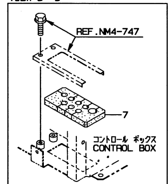
矢視 VIEW D-D
