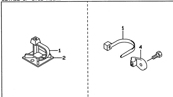
スタッド マウント 部群細 DETAIL OF STUD MOUNT
